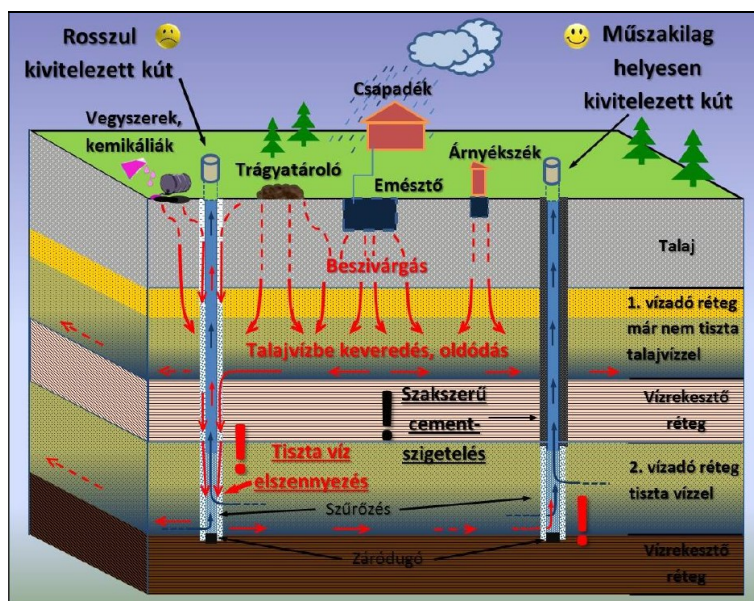
1. ábra Szakszerűtlen és szakszerű kút metszete és hatásai
